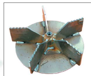
5 lopatek s pilovitým zakončením na rotoru násobí drtící a sací funkci
